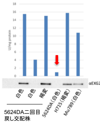
図1 β-1,3-グルカン分解活性 図2 各菌株の子実体
